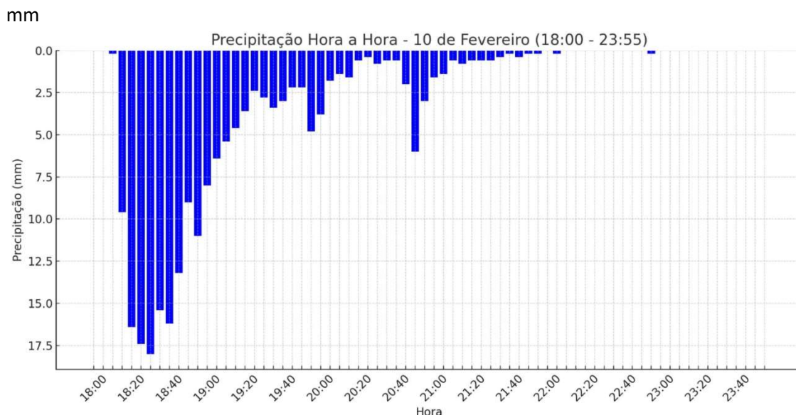
Figura 01. Precipitação em Cáceres no dia 10/02 entre às 18: e 23:55, totalizando 205.8
