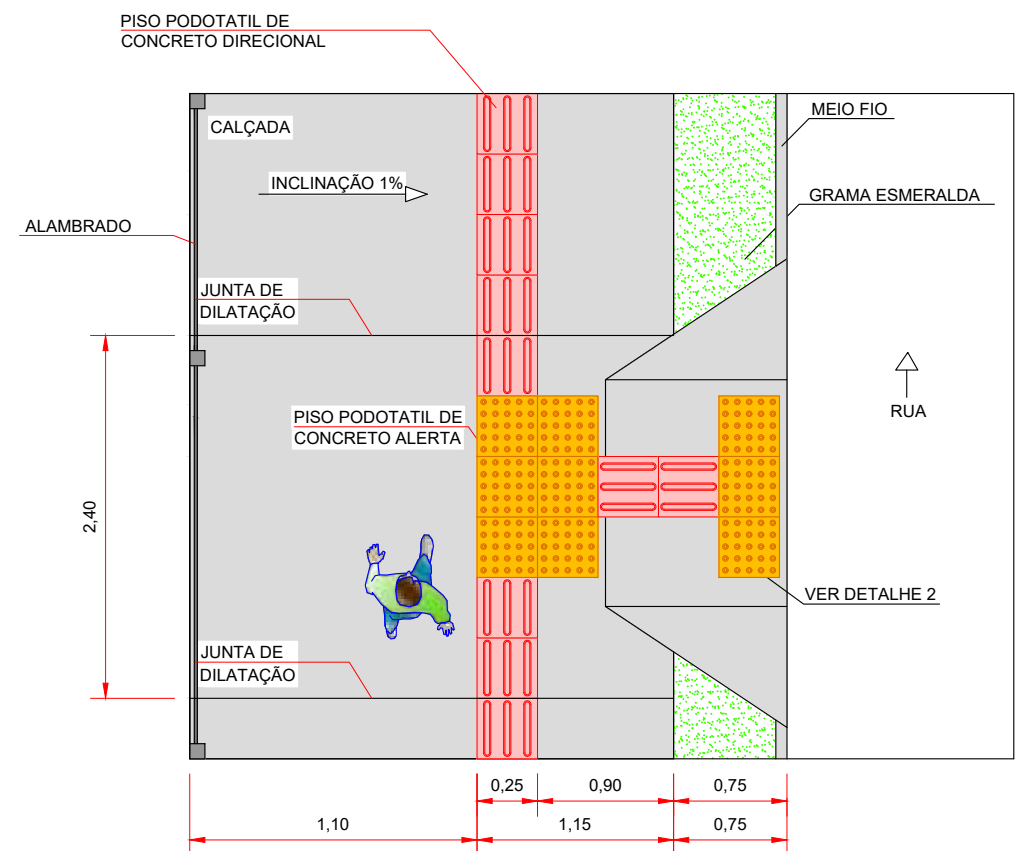
DETALHE CALÇADA FUNDO SEM ESCALA
