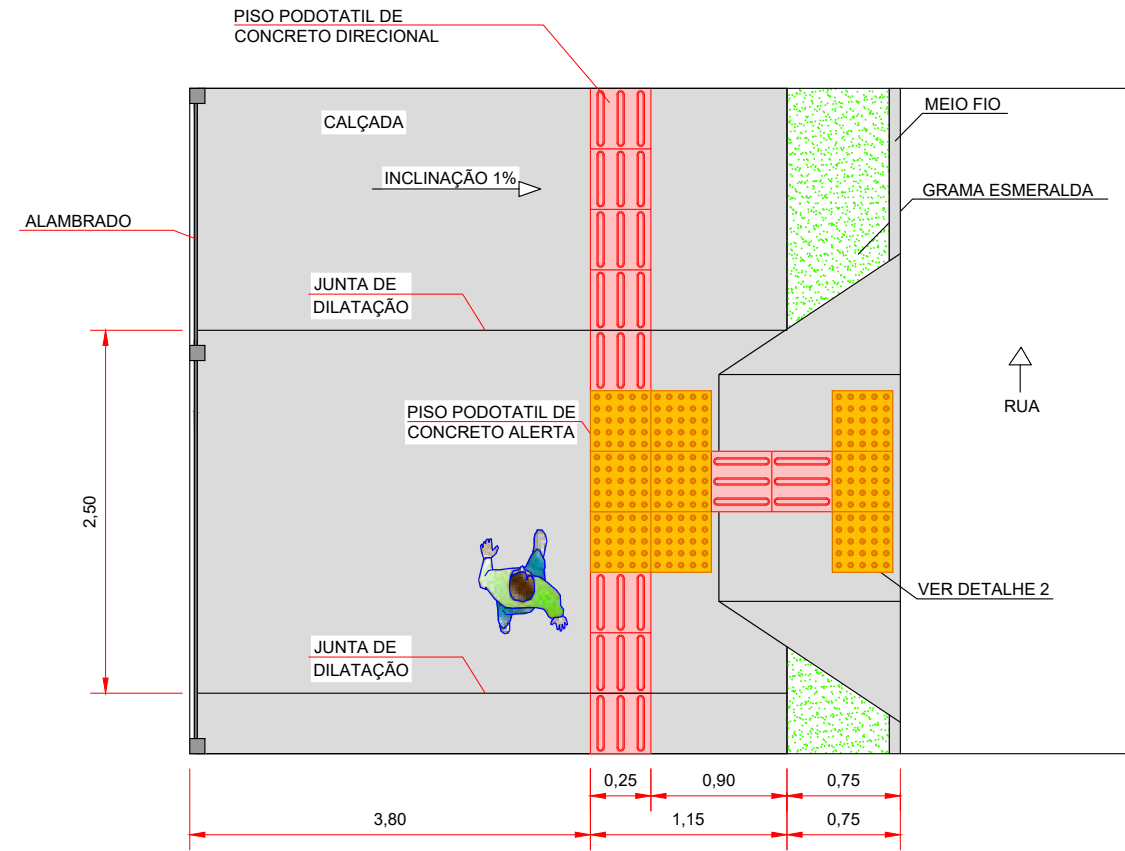
DETALHE CALÇADA FRONTAL SEM ESCALA
