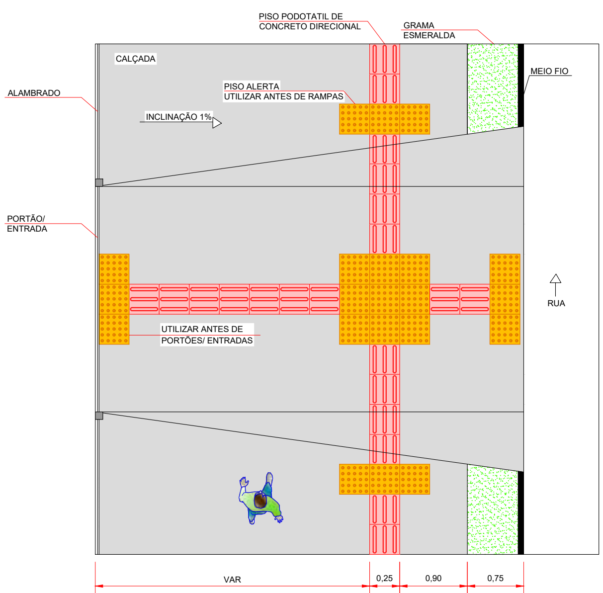
DETALHE 01 SEM ESCALA
