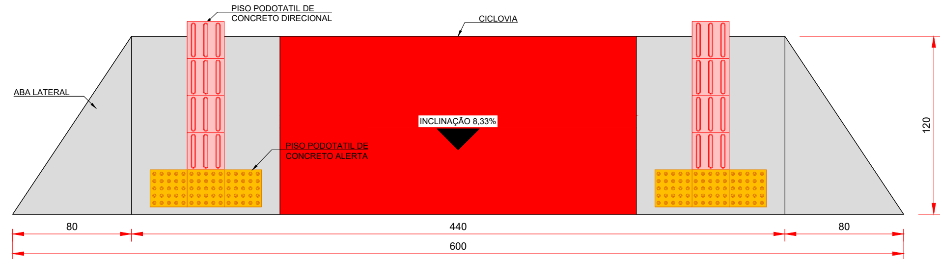
DETALHE 03 SEM ESCALA
