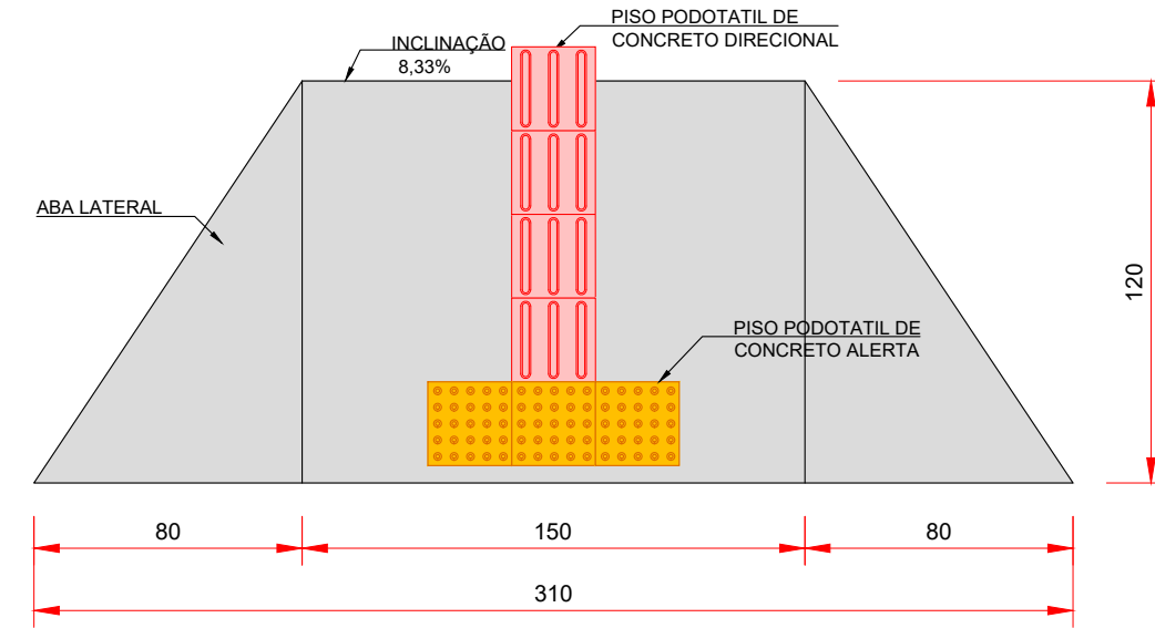
DETALHE 02 SEM ESCALA
