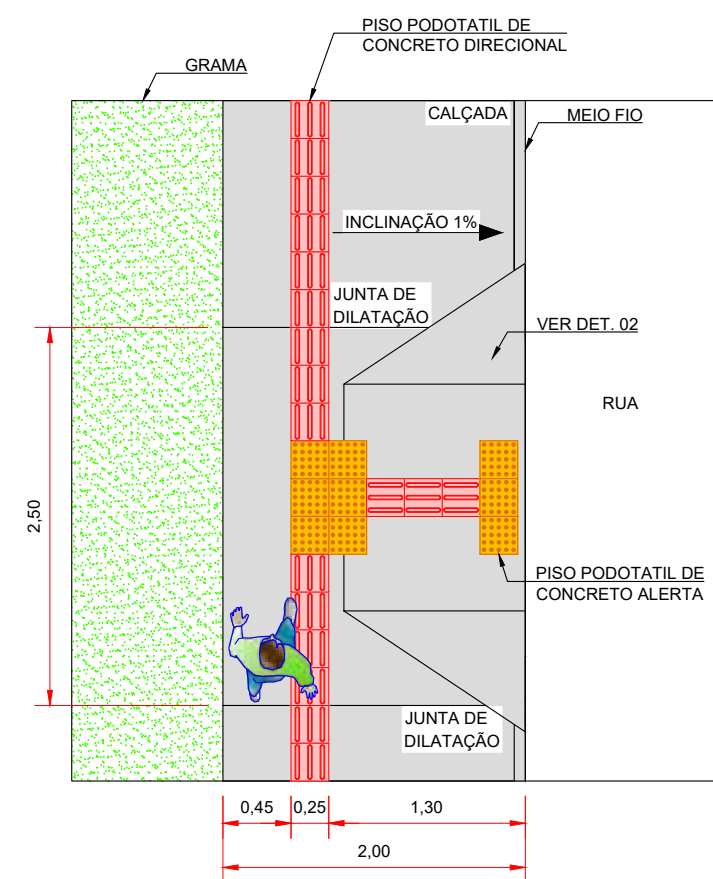
DETALHE CALÇADA SEM ESCALA
