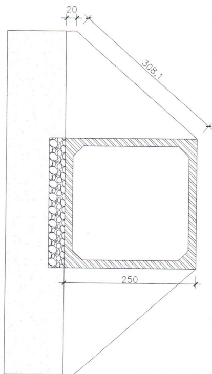
VISTA FRONTAL ESCALA 1:50
