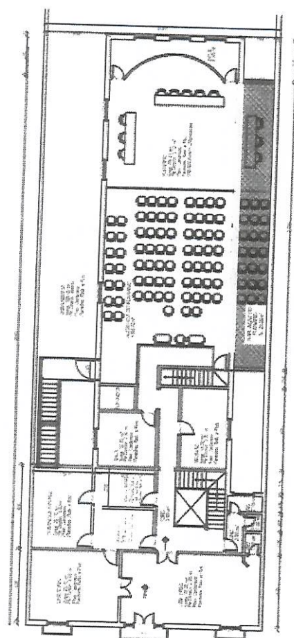
PLANTA BAIXA 2º PAVIMENTO
