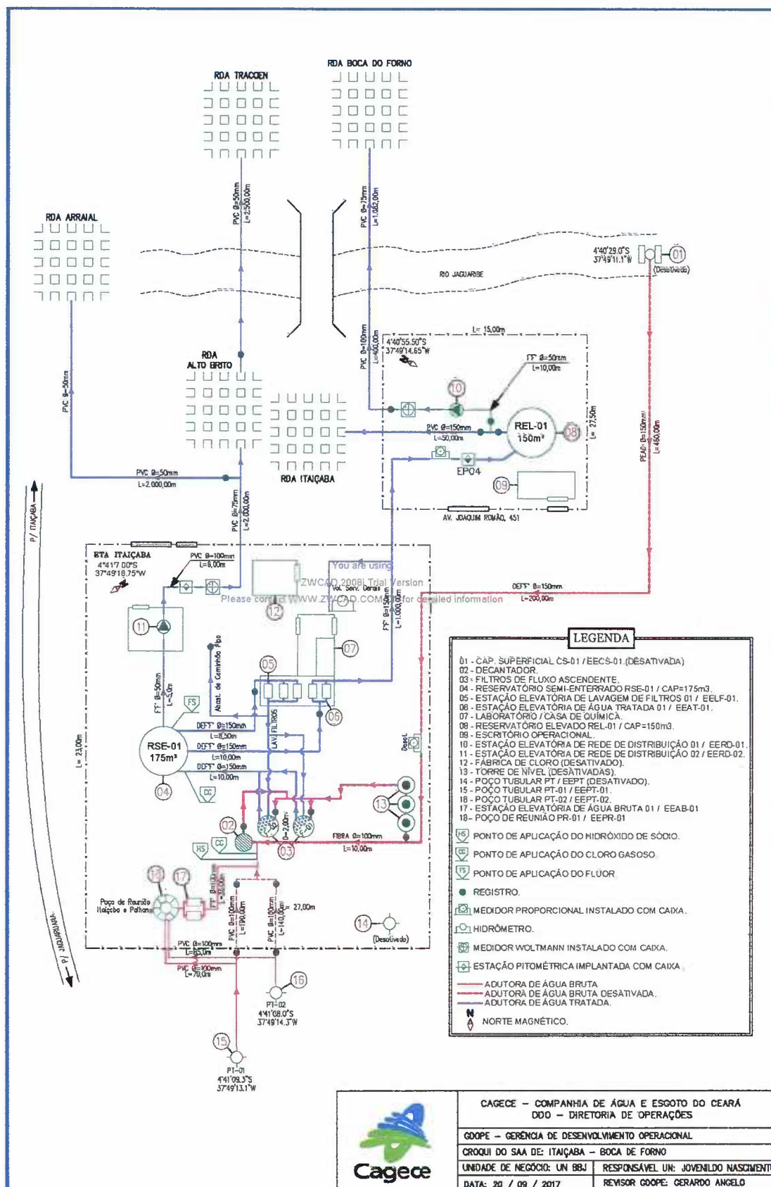
Figura 4.2 - Croqui do SAA da zona URBANA do Distrito Sede de Itaíçaba, 2018
