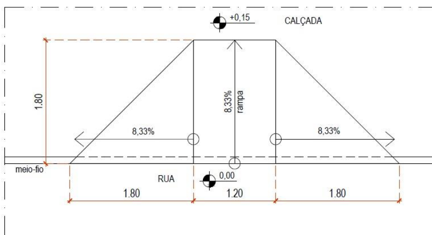
MODELO DE RAMPA DE PEDESTRES CONFORME NBR 9050/2015
