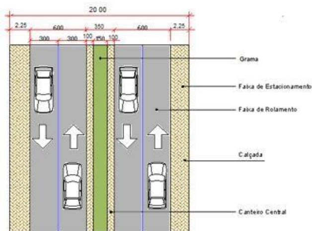
Planta Esquemática
