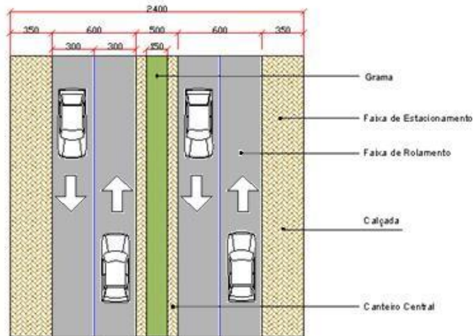
Planta Esquemática
