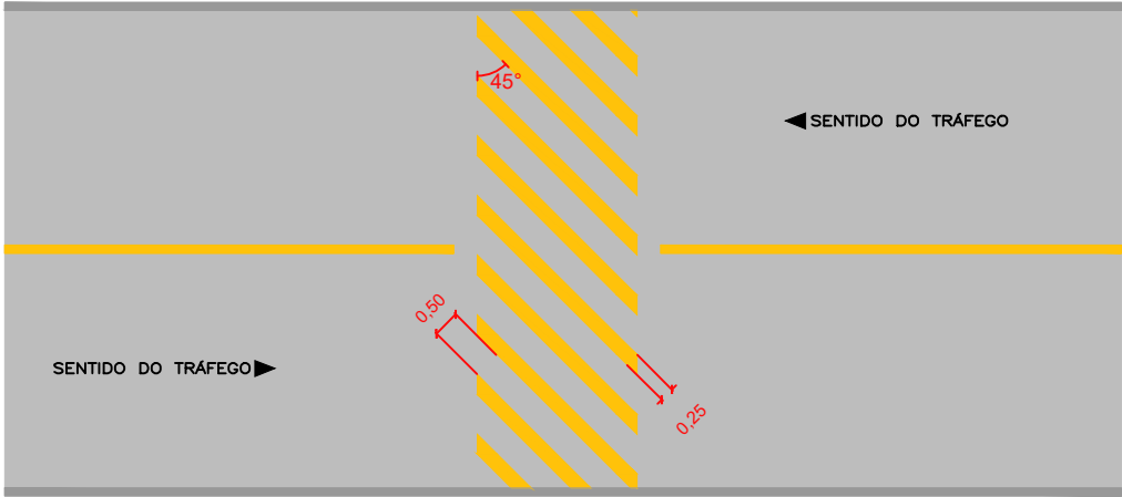
OT (ondulação transversal irregular)
