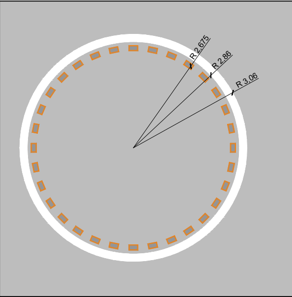
MINI ROTATÓRIA - NORMATIVA CONTRAN LOCALIZAÇÃO - RUA OSVALDO MERLIN C/ RUA ANTONIO AMORIM DE OLIVEIRA
