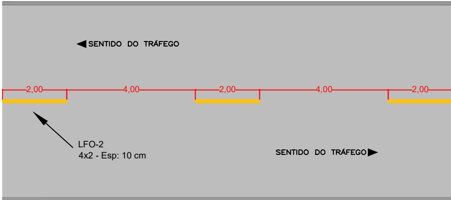
LFO-2 (fluxos opostos - simples seccionada)
