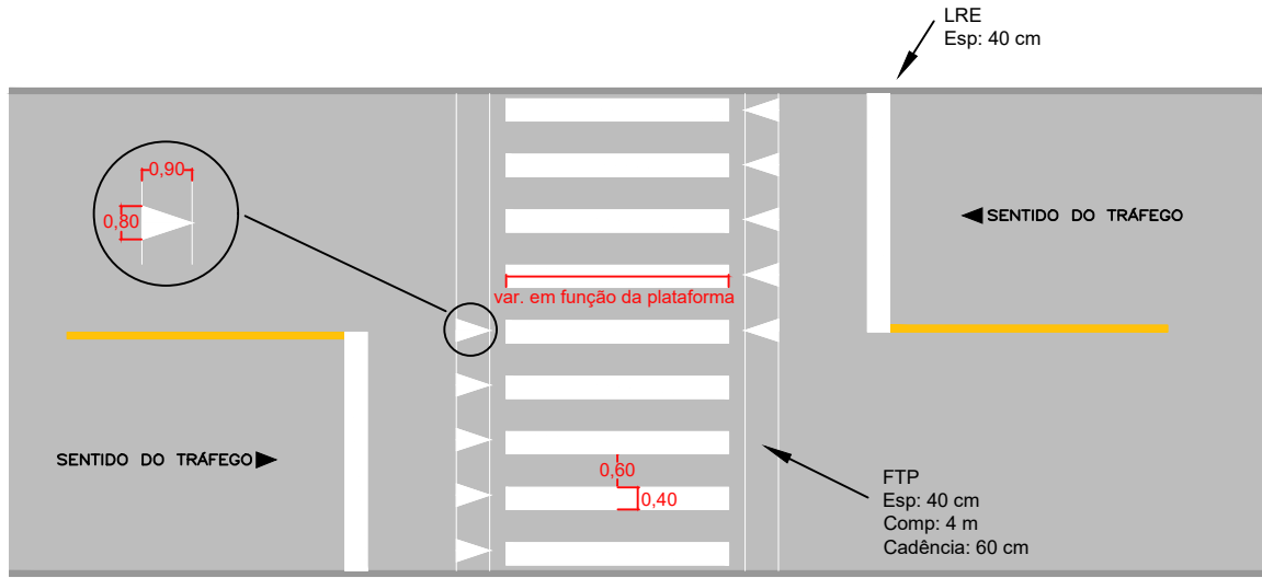
TE (travessia elevada)
