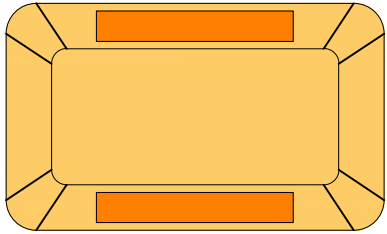
TACHÔES BIRREFLETIVOS: 15X25cm - ALTURA 5CM COR DO TACHÃO: AMARELO COR DO REFLETIVO: ALARANJADO
