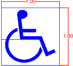
Símbolo "SIA" Dim: 1,00m x 1,00m Área: 0,15m² Azul: 0,85m²
