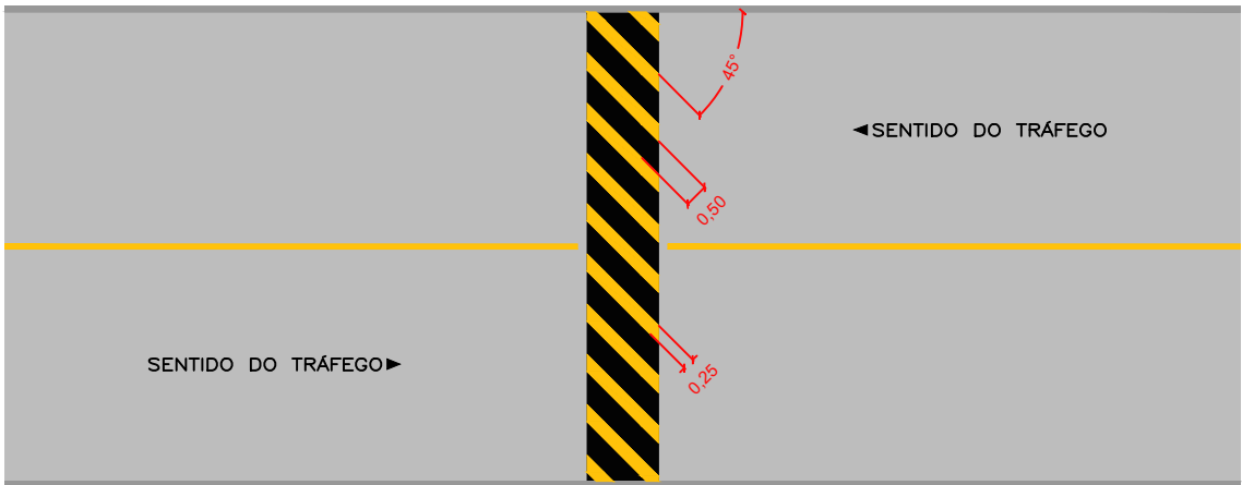
OT (ondulação transversal)
