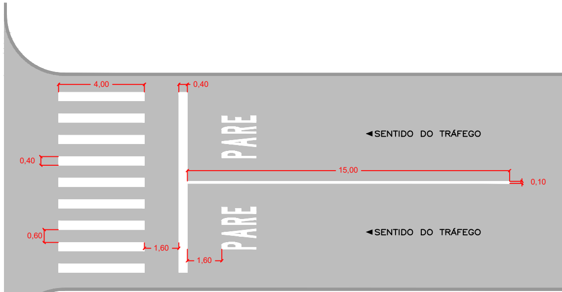
FTP/PARE (sentido único)
