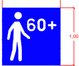
Símbolo "IDOSO" Dim: 1,00m x 1,00m Área: 0,18m² Azul: 0,82m²
