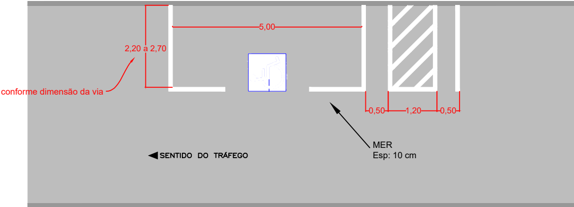
MER (estacionamento regulamentado)
