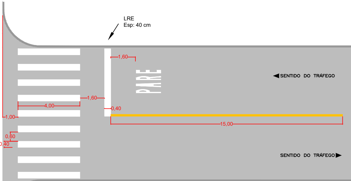
FTP/PARE (duplo sentido)
