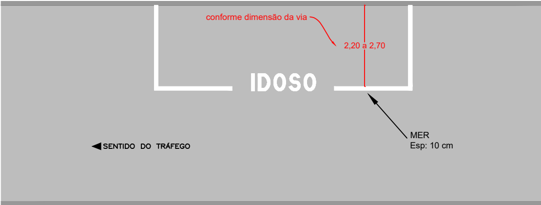
MER (estacionamento regulamentado)
