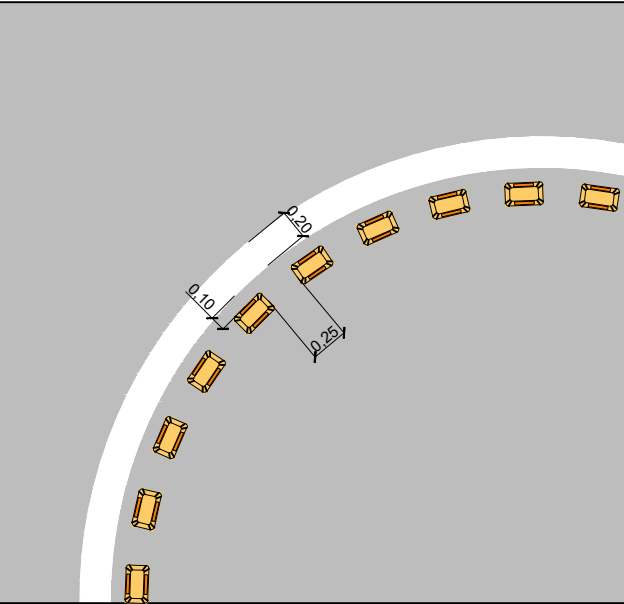
MINI ROTATÓRIA - NORMATIVA CONTRAN LOCALIZAÇÃO - RUA OSVALDO MERLIN C/ RUA ANTONIO AMORIM DE OLIVEIRA
