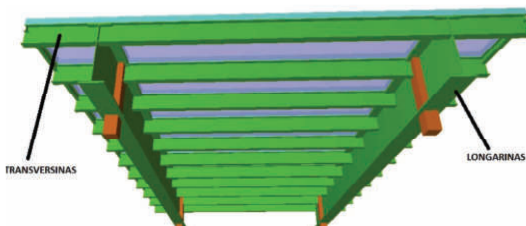
Imagem 5. Transversinas usadas em uma ponte mista
