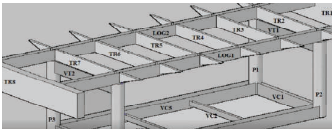
Imagem 6. Esquema de longarinas de reforço em ponte metálica
