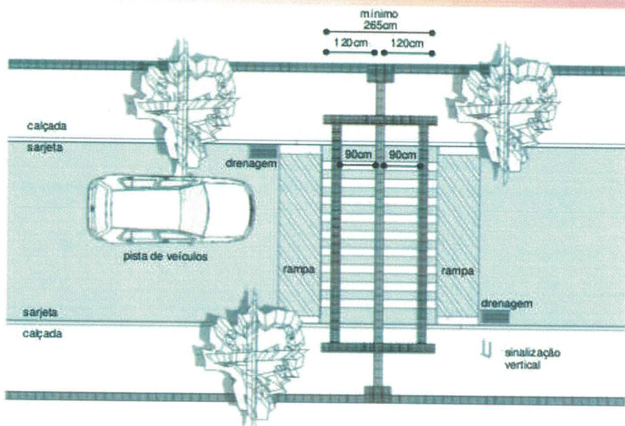
Figura 20 - Detalhe do piso tátil da passarela elevada
