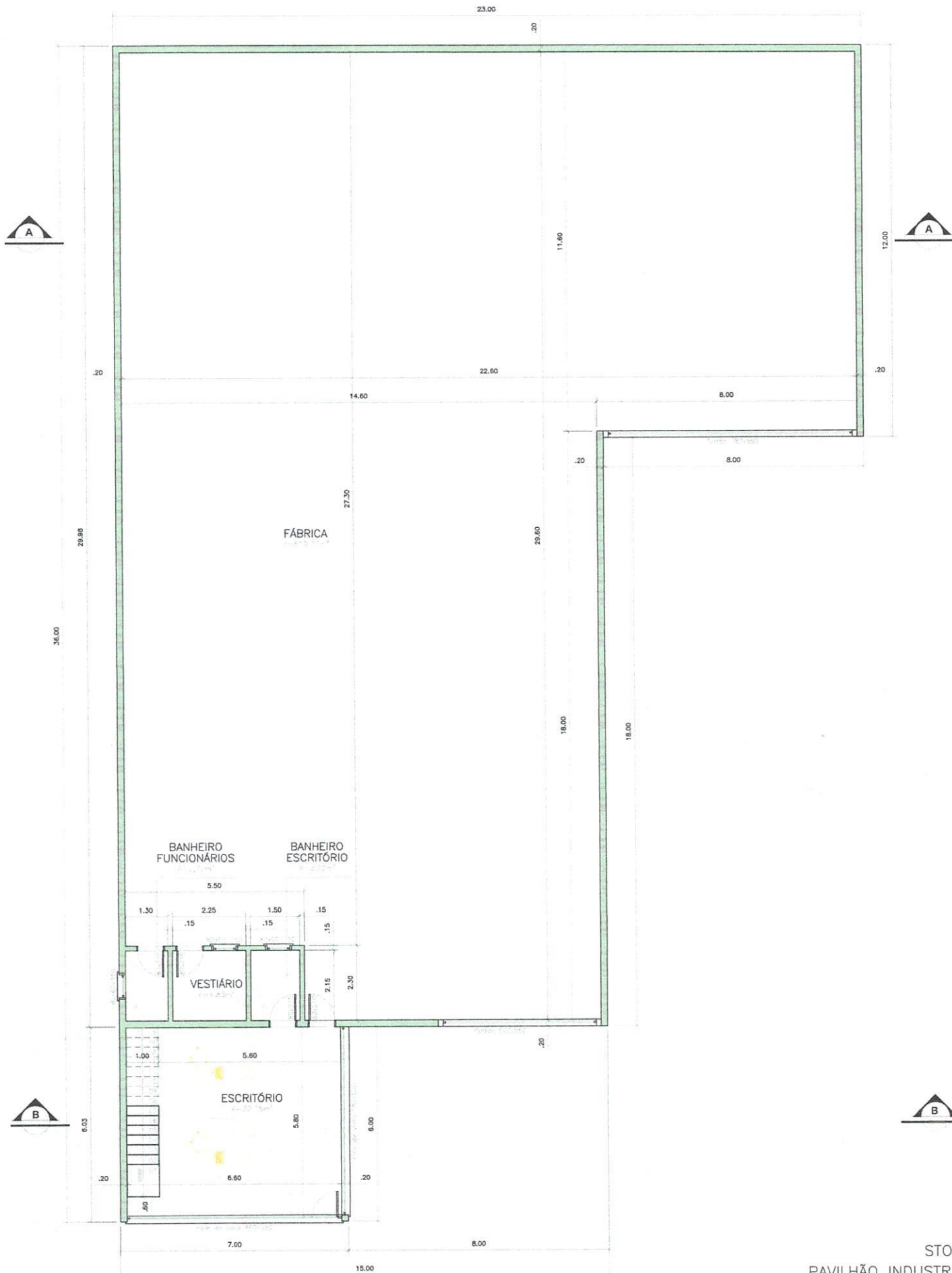
PLANTA BAIXA - TÉRREO PAVILHÃO INDUSTRIAL Área do pavilhão: 696,30m² Área do terreno: 1.217m²
