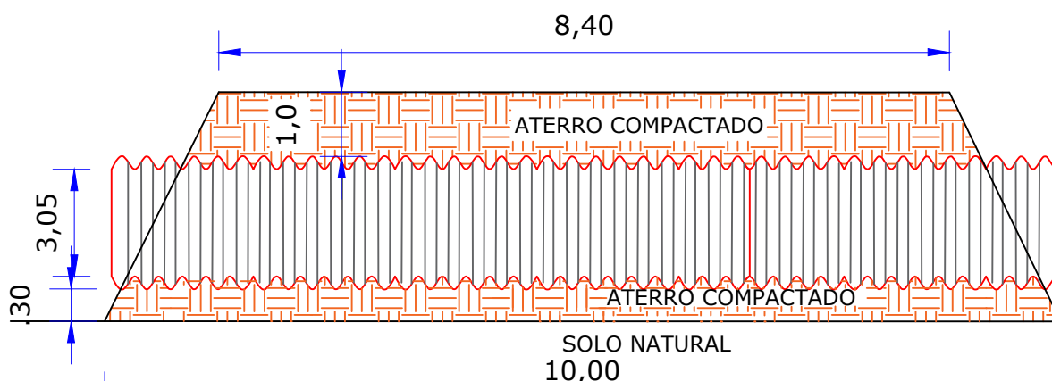
CORTE AA - PONTO 01 ESC: Sem ESC.
