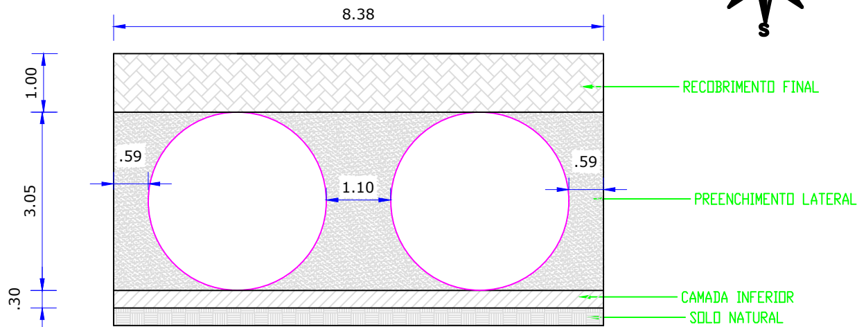
CORTE BB - DUPLO -PONTO 01 ESC: Sem ESC.
