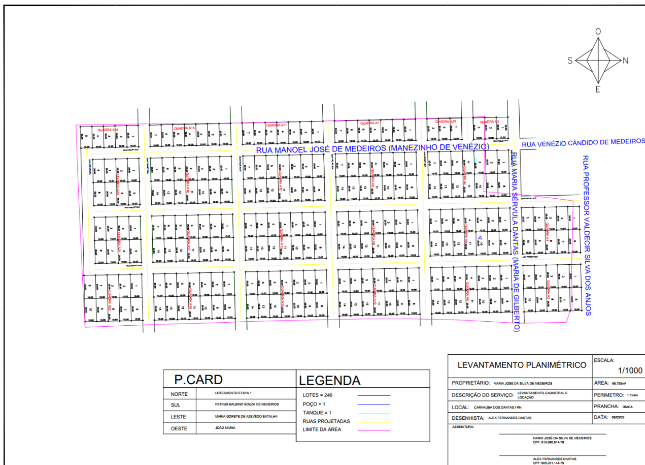
Foto 2: Planta planimétrica do Loteamento Etapa 2, contendo a divisão de quadras, lotes e vias projetadas, localizado na Rua Maria Sérvula Dantas (Maria de Gilberto), no Município de Carnaúba dos Dantas/RN.
