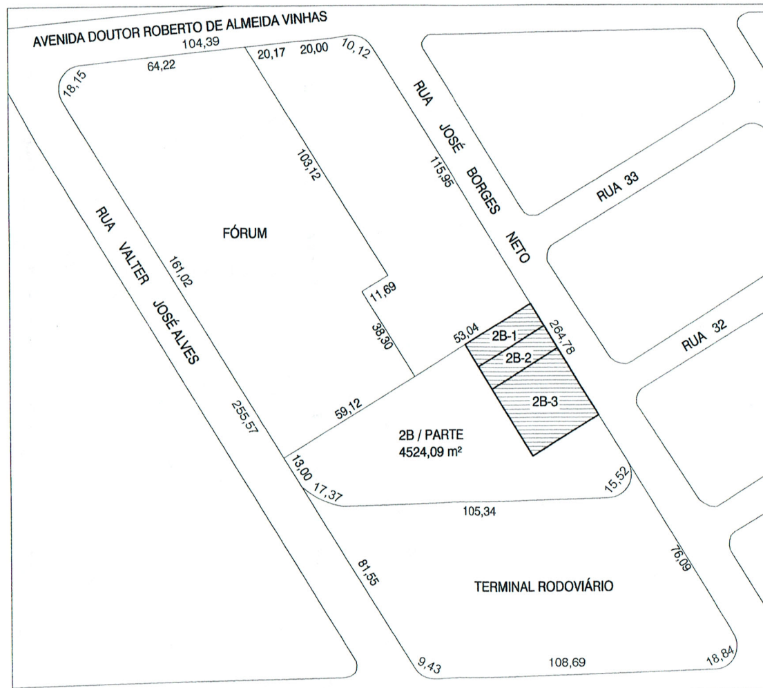
01 LOCALIZAÇÃO 1:2000
