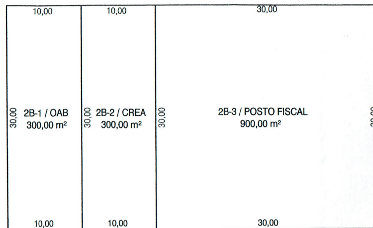
03 ÁREAS 1:500
