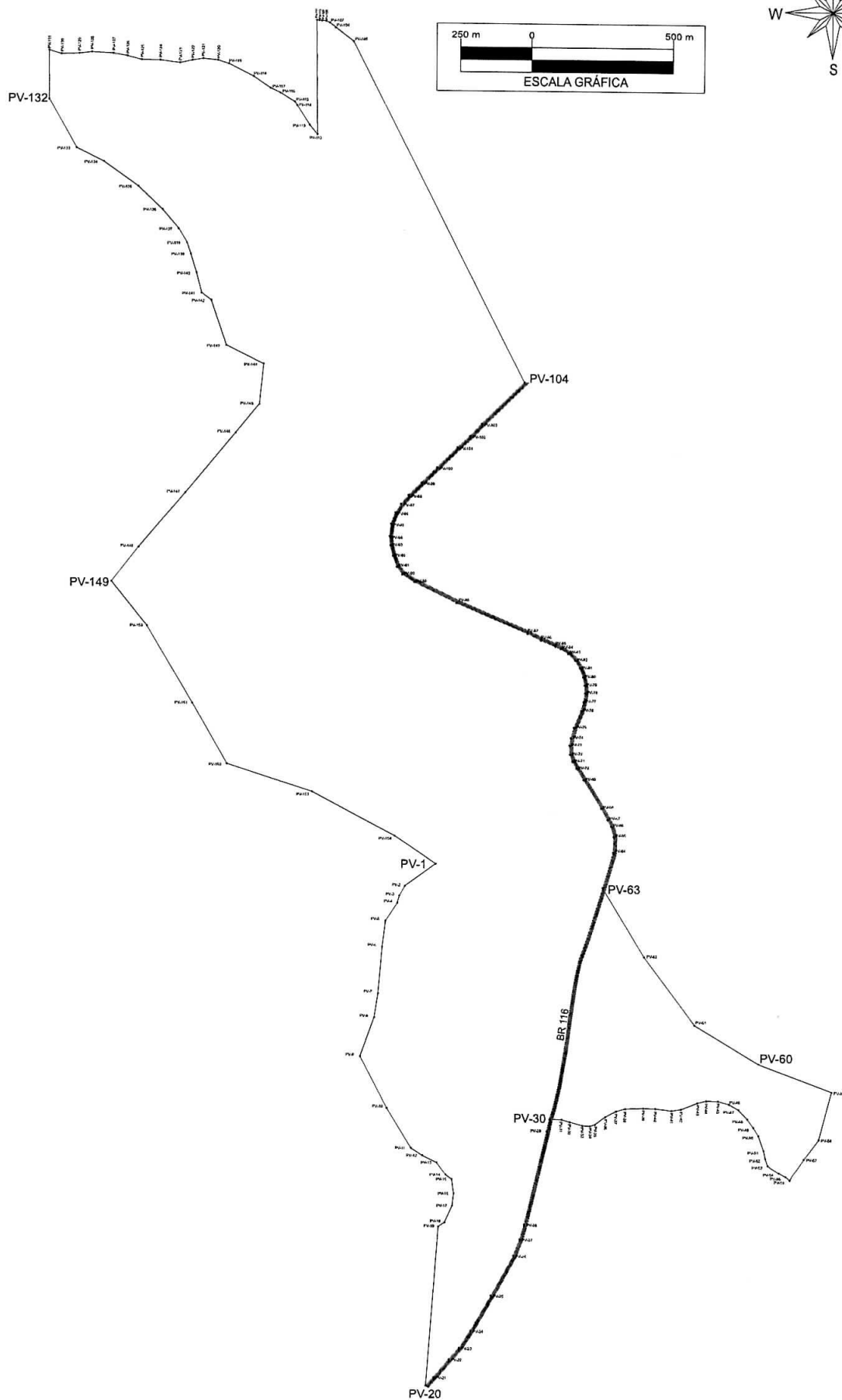
PERÍMETRO URBANO DO DISTRITO DE ITAMURI ESCALA: 1:20.000
