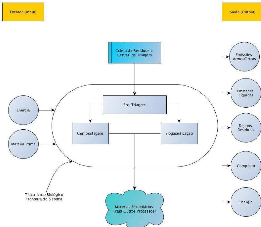
Figura 3.2 - Tratamento Biológico e Seus Processos.
