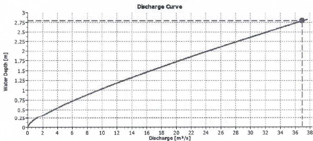
Figura 7 - Curva Cota x Vazão para a seção transversal da travessia projetada
