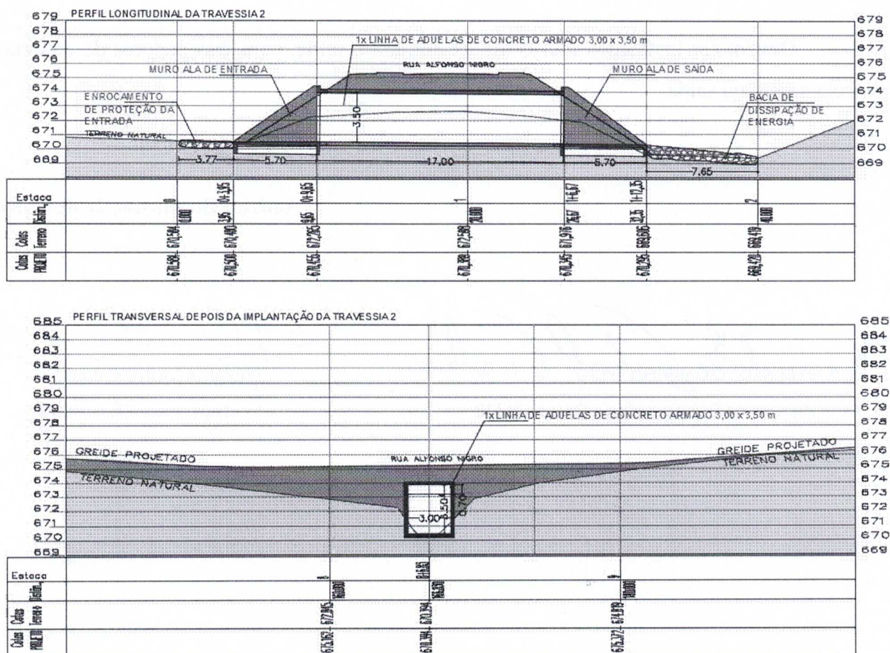
Figura 9 - Esquema da nova travessia
