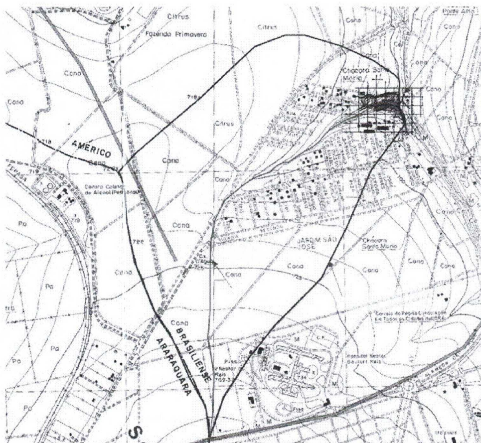
Figura 3 - Bacia de contribuição à seção de entrada da Travessia 2 sobre o afluente do Córrego da Ponte Alta.
