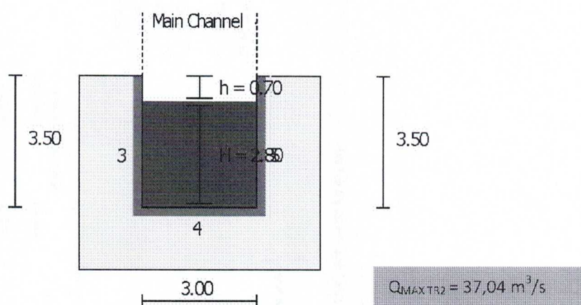
Figura 6 - Esquema hidráulico considerando-se a capacidade máxima na Travessia 2.
