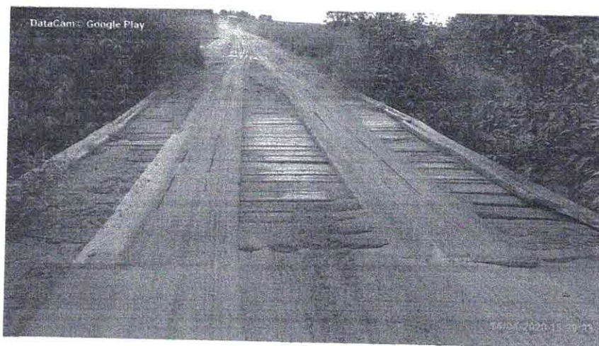
Figura 10: Vista superior da ponte.
